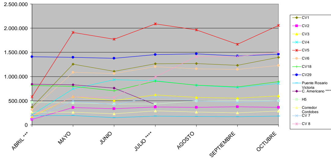
TRÁNSITO TOTAL MENSUAL CORREDORES VIALES AÑO 2010 Abril a Octubre
